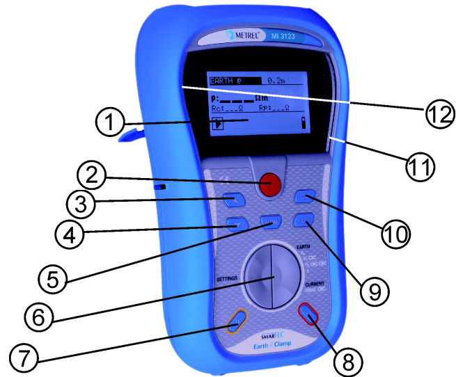
Face avant du contrôleur
